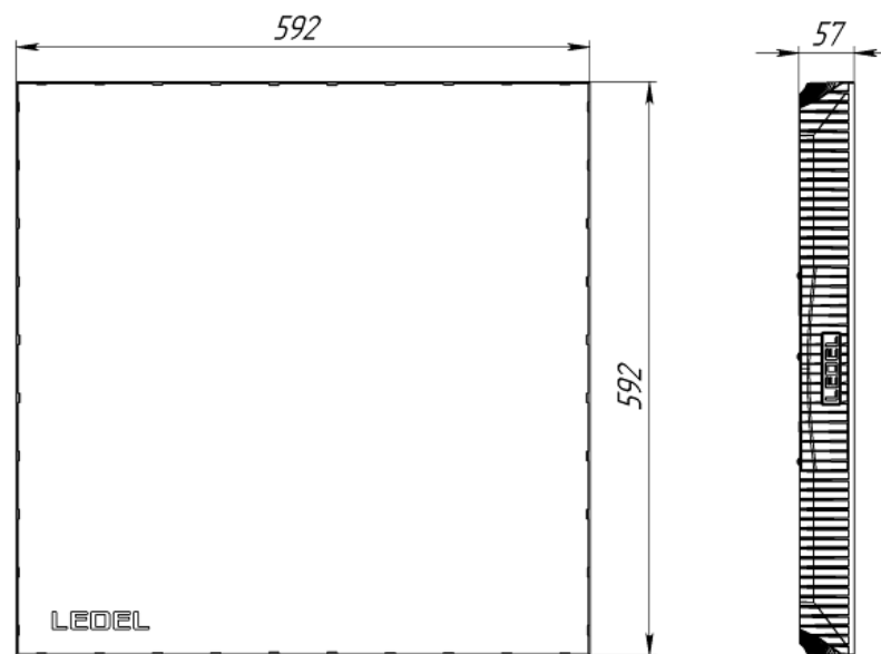
Рисунок 1 Светильник «L-office 32 Standart», «L-office 55 Standart»
